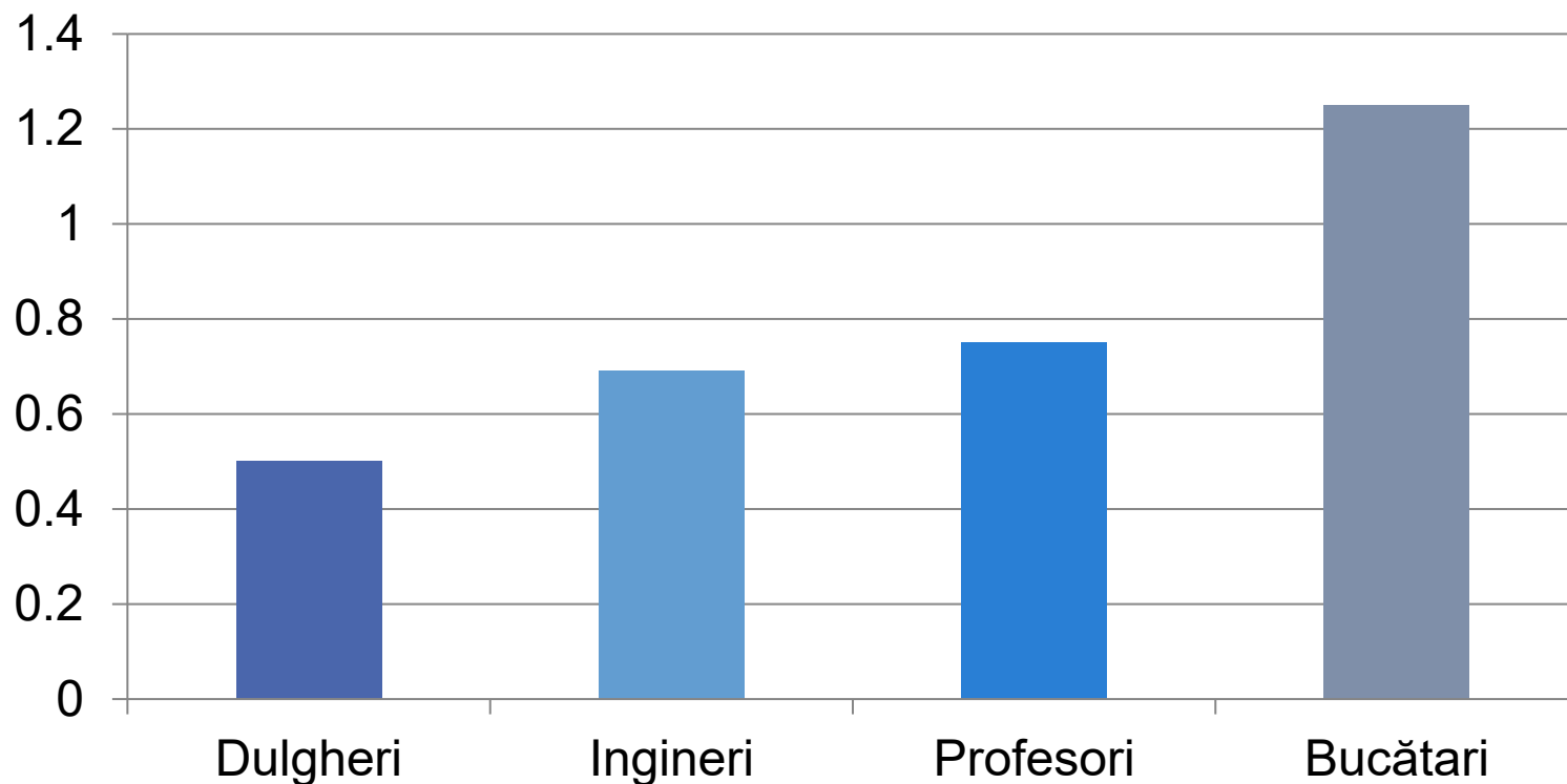
Rata de incongruență
